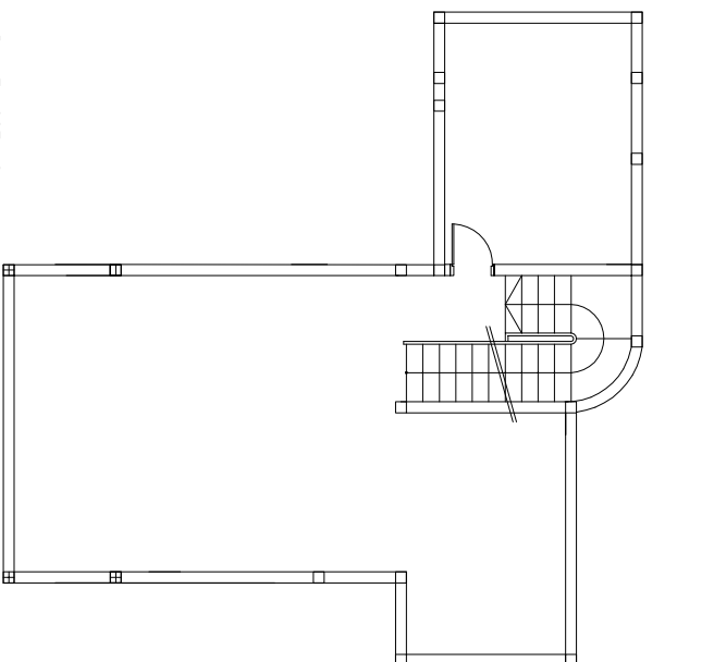
PLANTA SOTANO T3-17.50
