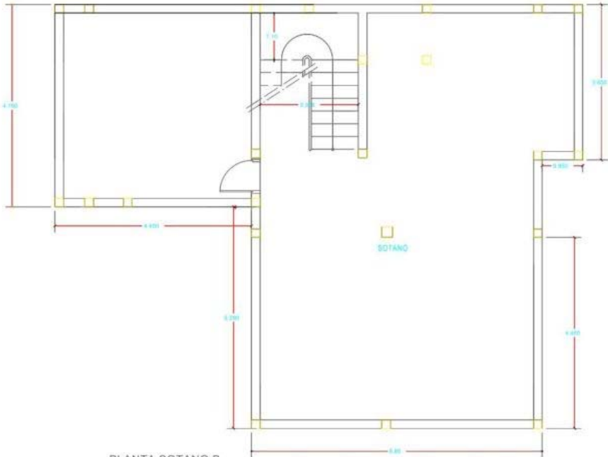
PLANTA SOTANO B
